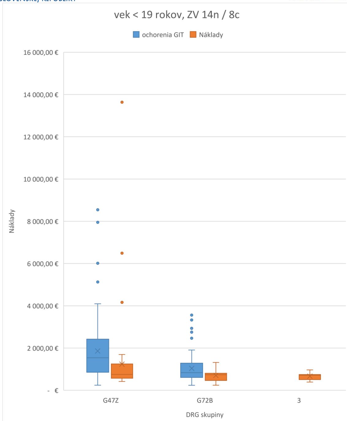
Graf 1: Grafické zobrazenie nákladovosti hospitalizačných prípadov (HP) s vykázanými ZV 14.11.2, 14n11.2 (ozn. 14n) alebo ZV 8c105 – 8c108 (ozn. 8c) s rôznymi hlavnými diagnózami – ochorenia GIT (modrá), T18.- (oranžová) zaradených do DRG G47Z, G72A (ozn. 3) alebo G72B.
