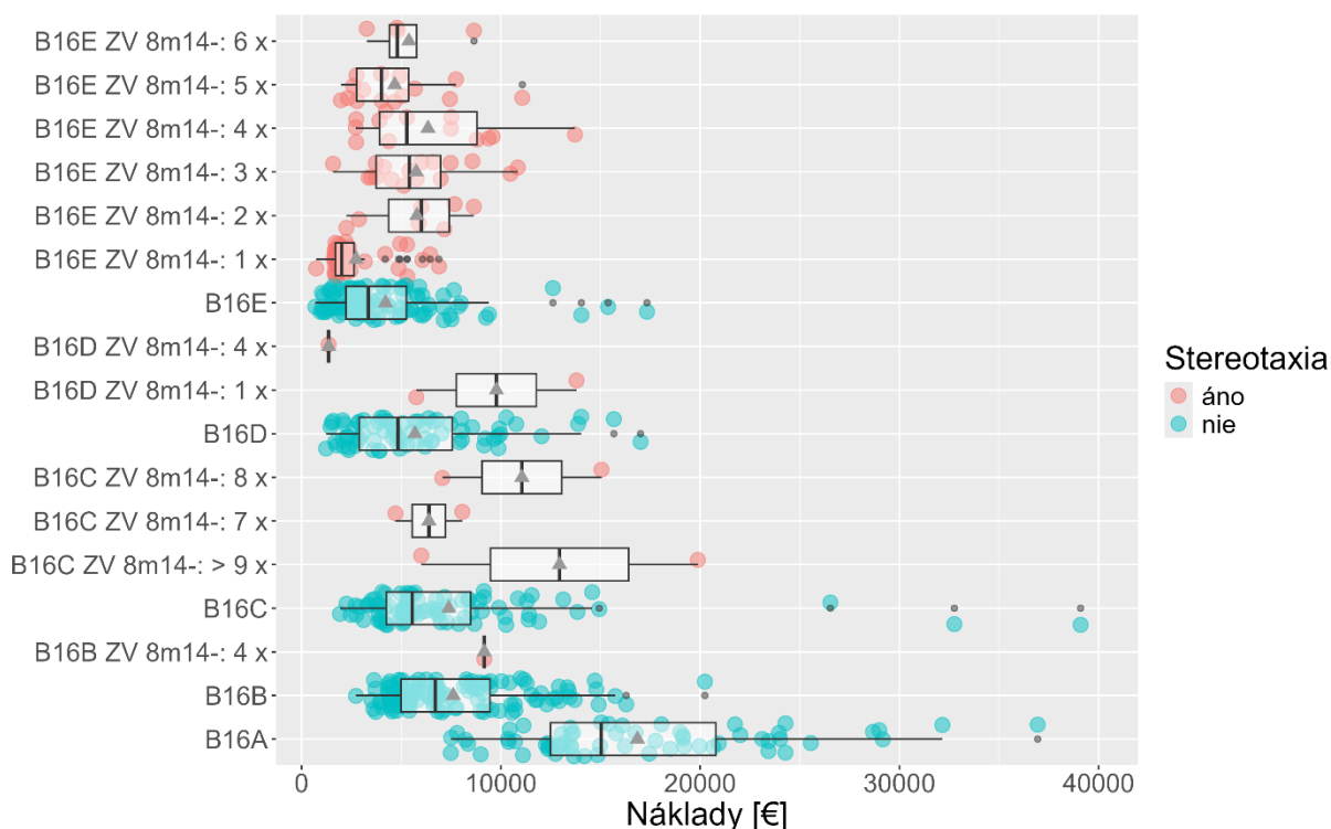
Graf 6 Rozloženie nákladov prípadov podľa DRG skupiny a počtu vykázaných výkonov 8m14- v pôvodnom návrhu (verzia 2)
