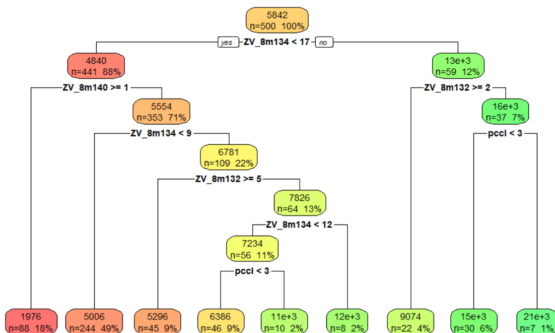
Obrázok 1 Príklad rozhodovacieho stromu vytvoreného rpart modelom pre ADRG B15 a B16
